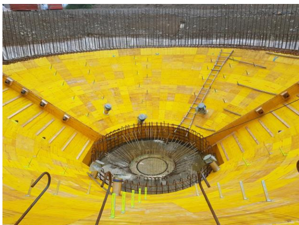
Coffrage digesteur
